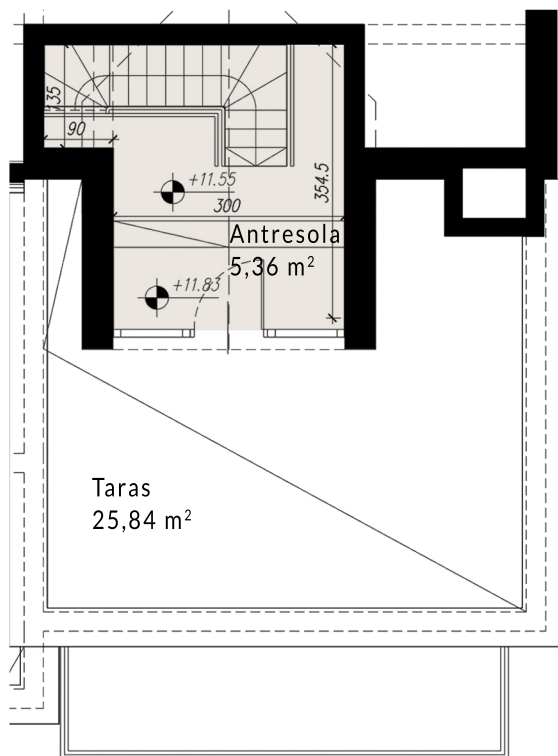
RZUT ANTRESOLI
