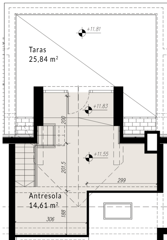
RZUT ANTRESOLI
