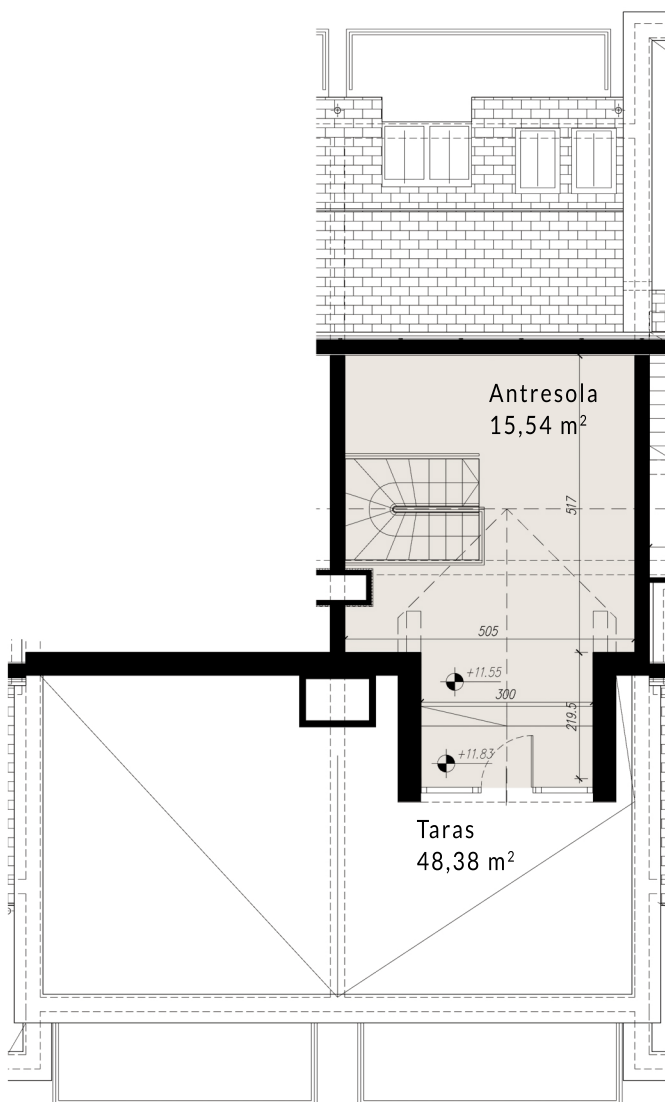
RZUT ANTRESOLI
