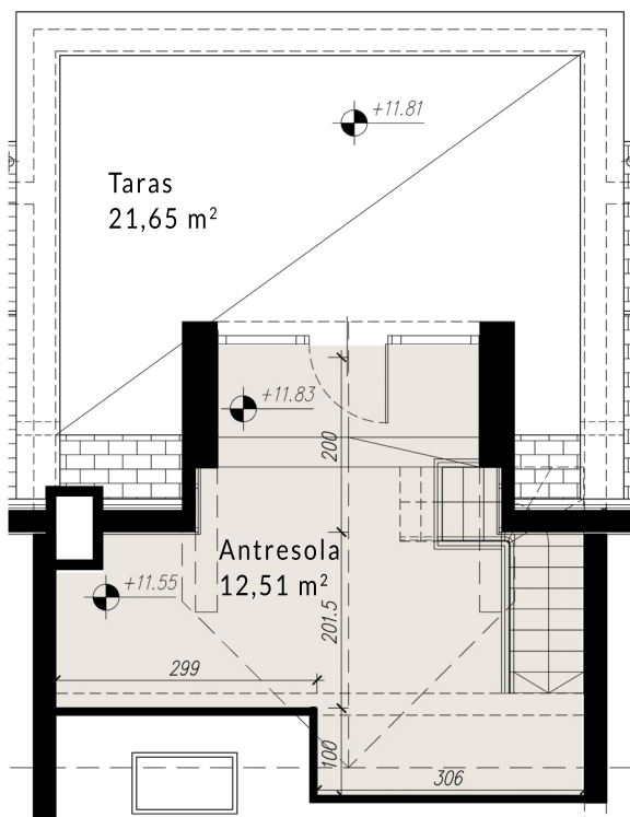
RZUT ANTRESOLI
