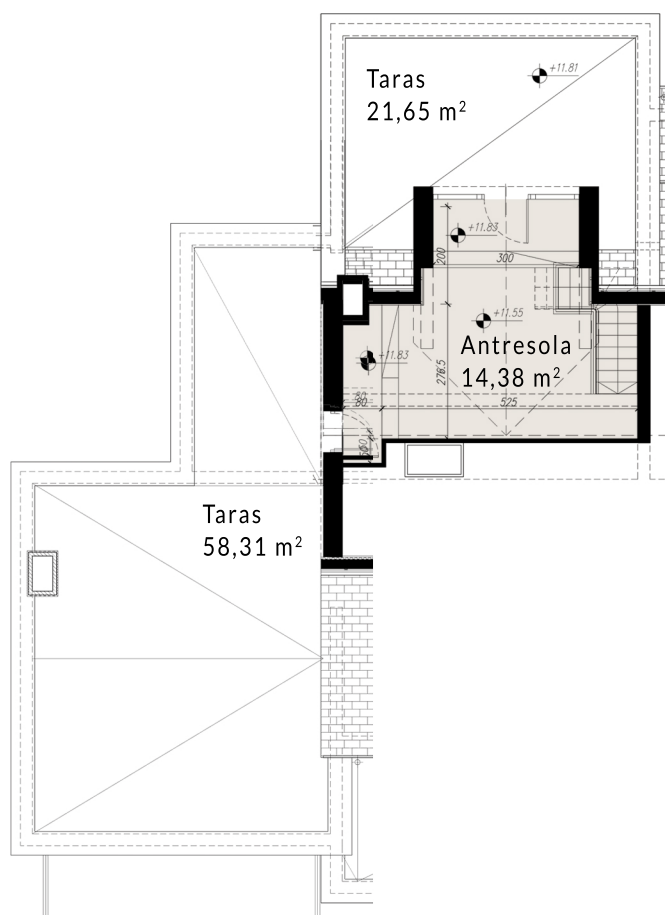
RZUT ANTRESOLI
